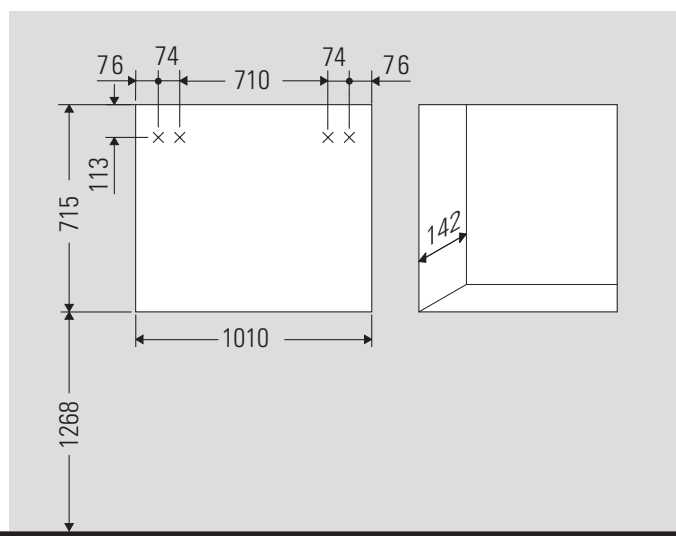
Dimension de découpe pour les meubles encastrés
